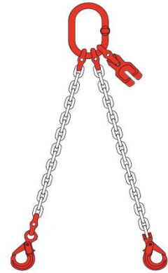
MONTAGE AVEC CROCHET À CHAPE ET RACCOURCISSEUR
