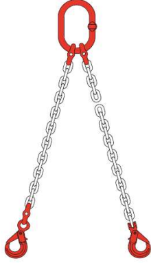
MONTAGE AVEC CROCHET À OEIL
